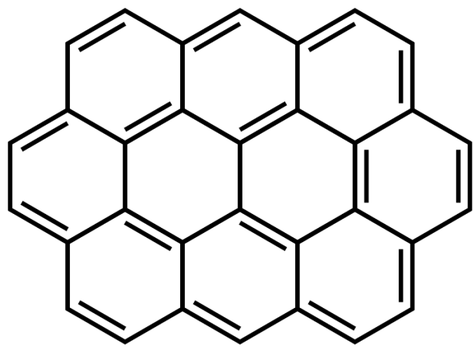
Ovalén
