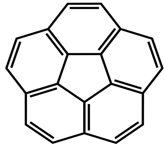
Korannulén
