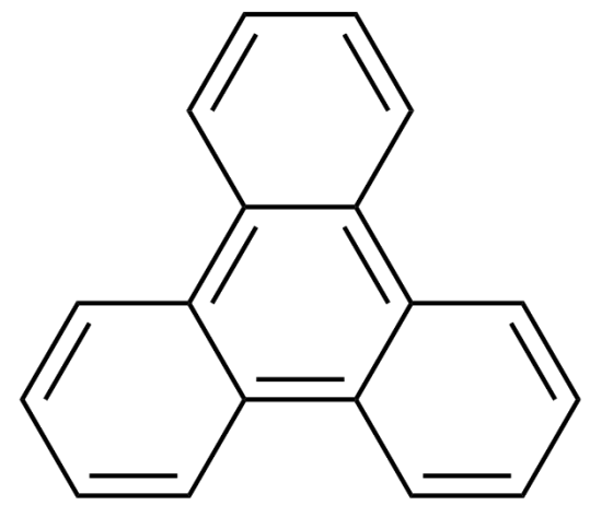
Trifenilén
