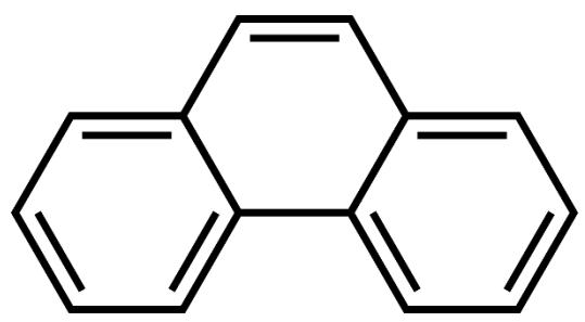
Fenantrén
