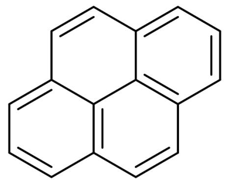
Pirén
