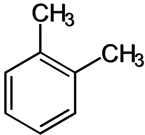
1,2-Dimetilbenzol
