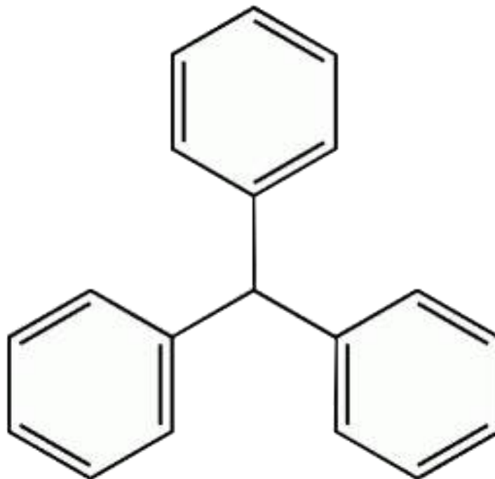
Trifenilmetán
